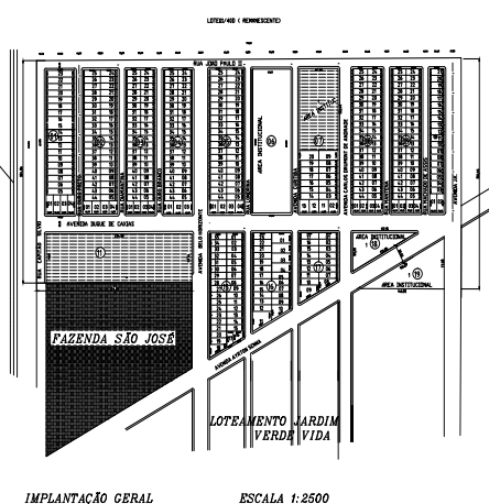
IMPLANTAÇÃO GERAL ESCALA 1:2500
